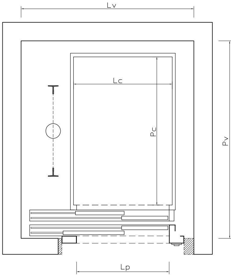
PIANTA VANO
