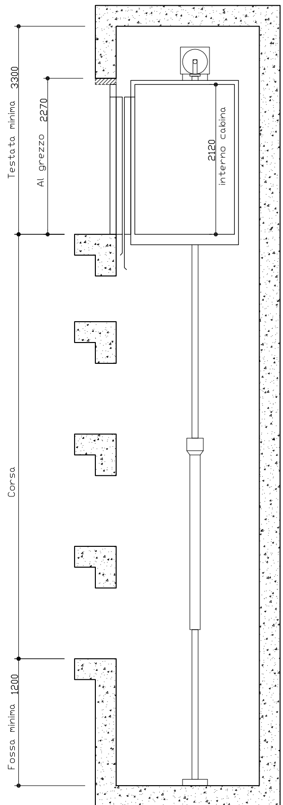
SEZIONE VERTICALE
